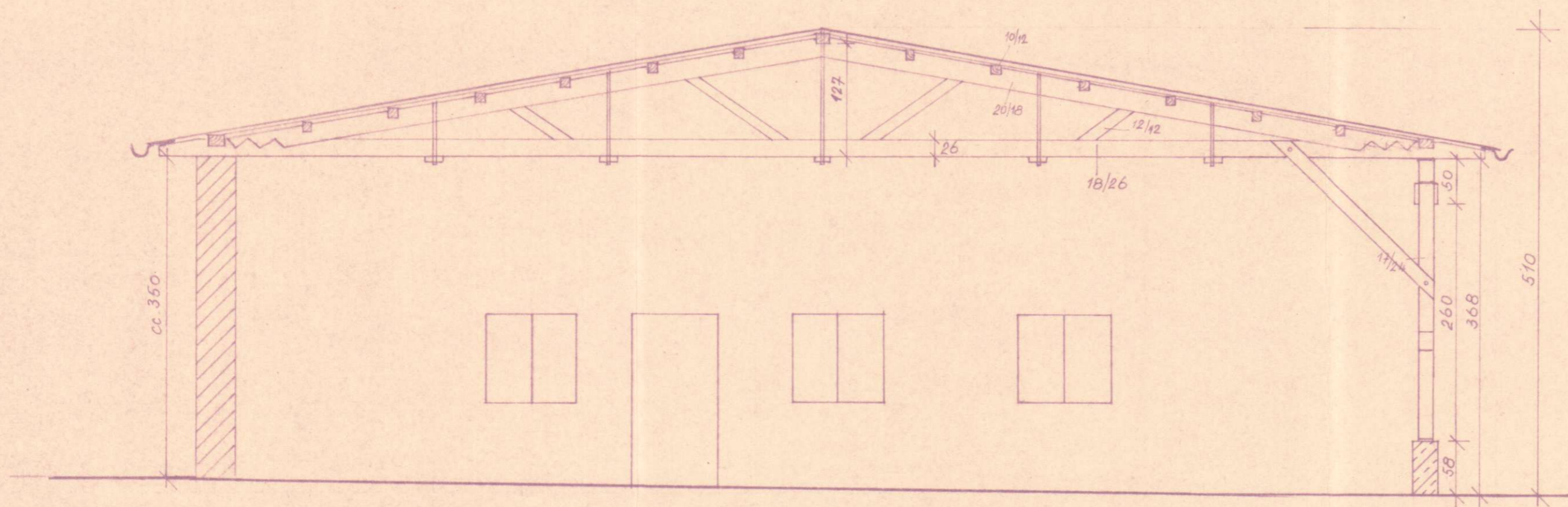
PREREZ A-A
